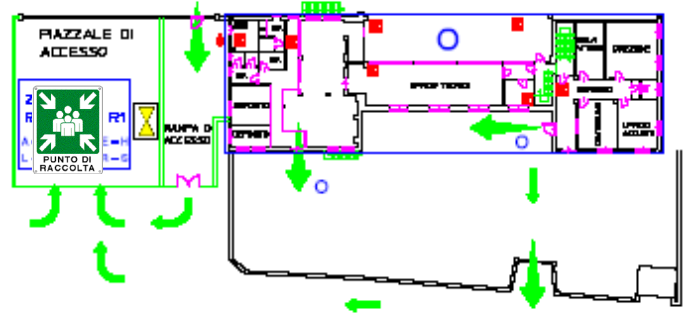
PIANO DI EMERGENZA UFFICI | PIANO TERRENO
